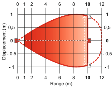
CDR-RED2.0 16 canali
