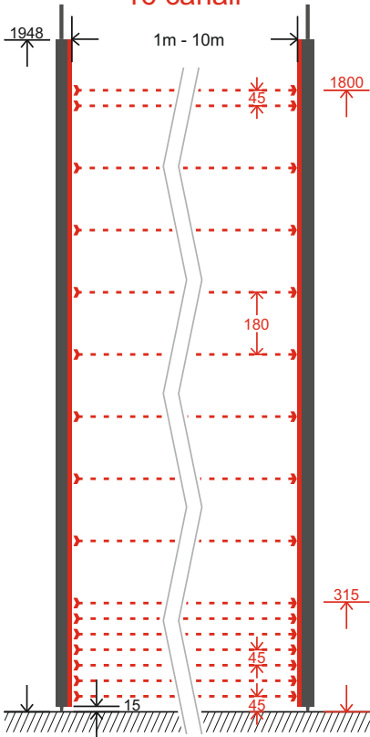
CDR-RED2.0 16 canali
