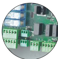
MORSETTIERE ESTRAIBILI
