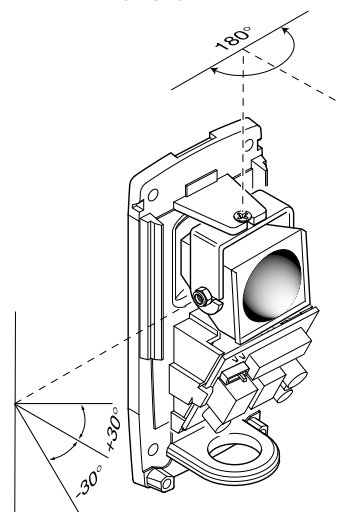
OTTICA ORIENTABILE
