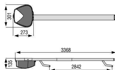
GLZEN60E - GLZEN100E
