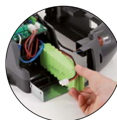
OPZIONE BATTERIE NIMH
